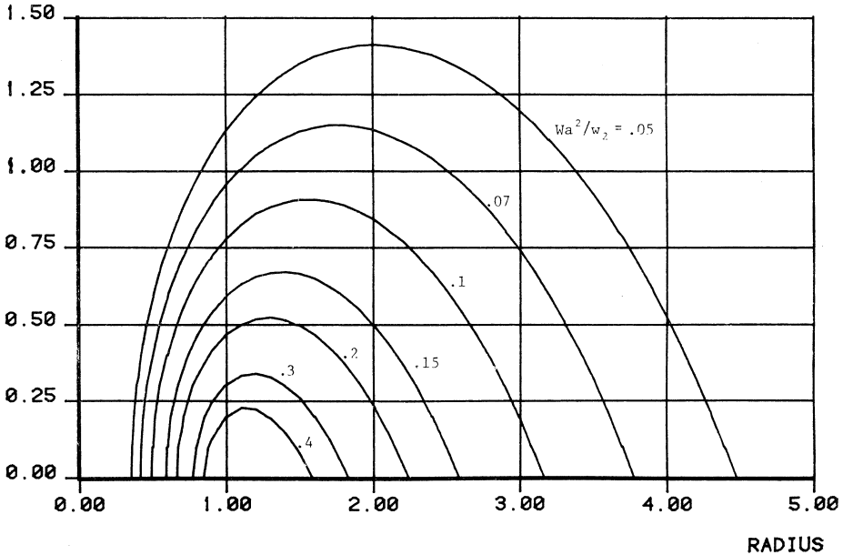
Fig. 3. Equipotential lines for n = 2
