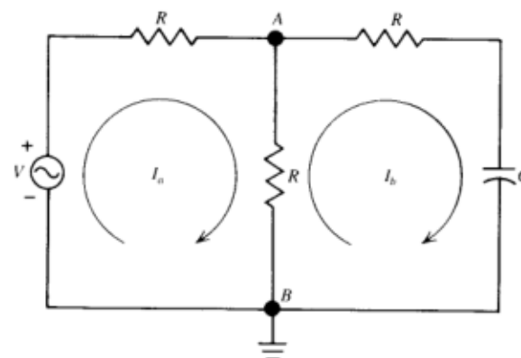
Fig. 7-16. Simple RC circuit.
