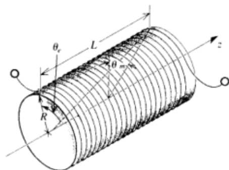
Fig. 18-5. Solenoid.
