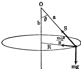
FIG. 135.—Conical pendulum.
