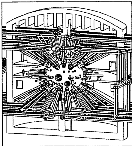
(b) NIF DD beam geometry
