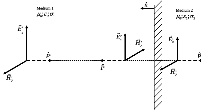
Figure 4.1: Poner los valores de pynting \mathcal{P} El subindice de campo electrico incidente ponerlo mejor
